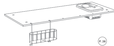
PRO BAR TOP L71" W29.5" | L180cm W75cm Ice Bin: L16" W9" D6" L41.5cm W23cm D15cm
