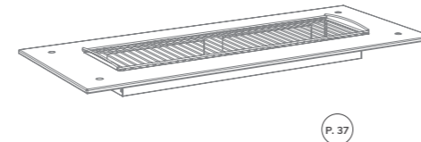
HEAT TABLETOP L71" W29.5" | L180cm W75cm Grill: L48" W25" D6.5" L122cm W63cm D16cm
